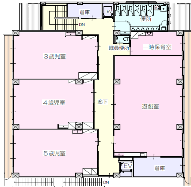
2階平面図
